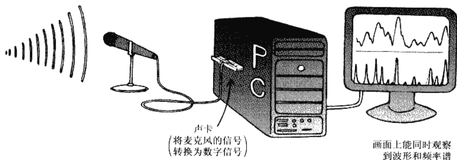
◆图7.6 利用电脑观察声音的波形
