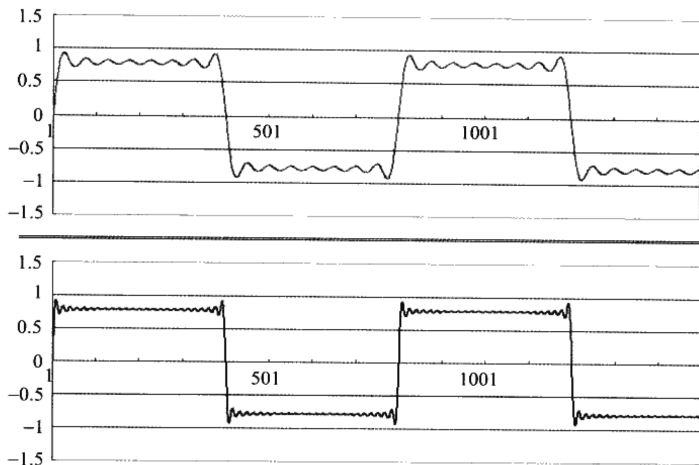
◆图 6.16 n = 15 时累加合成的波形(上)与 n = 49 时累加合成的波形(下)
