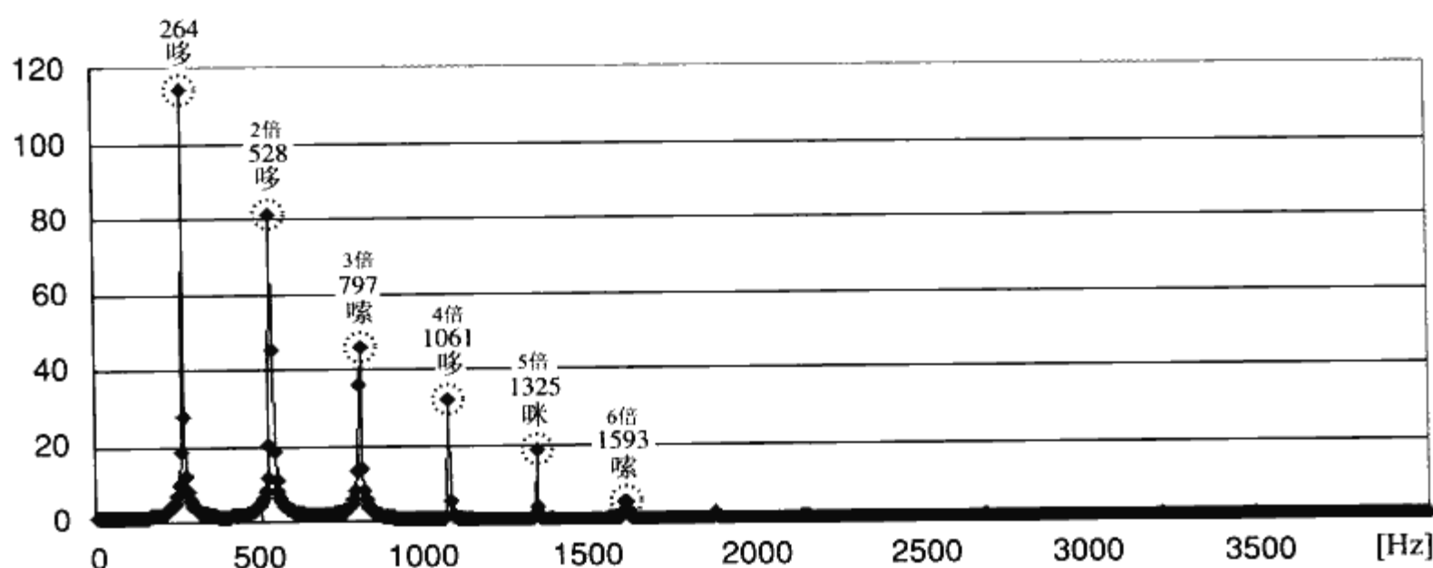
◆图 7.11 “哆 C”音的频率谱中的主要峰值的频率
