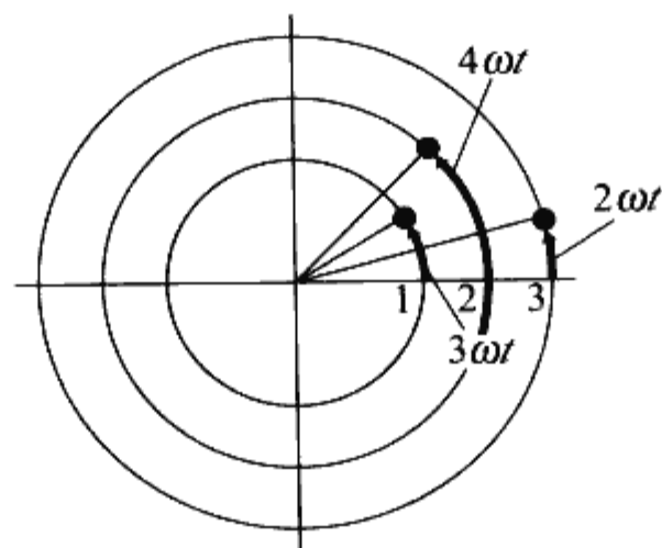
◆图6.17 分别在三个圆周上旋转的点
