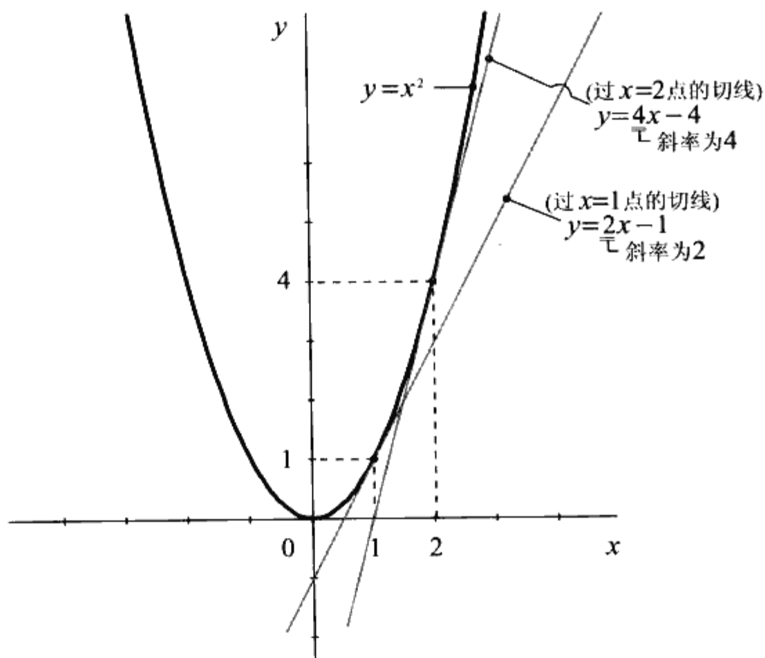
◆图 3.13 y = x^2 切线的斜率
