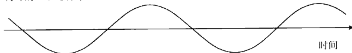
◆图1.5 在波浪中晃动的树叶随时间变化的运动
