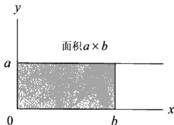
◆图3.1 y=a 、 x=b 代入微分公式
