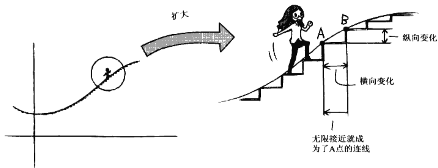
◆图 3.11 关于台阶的斜率：B 无限接近 A，AB 直线就会变成过 A 点的切线
