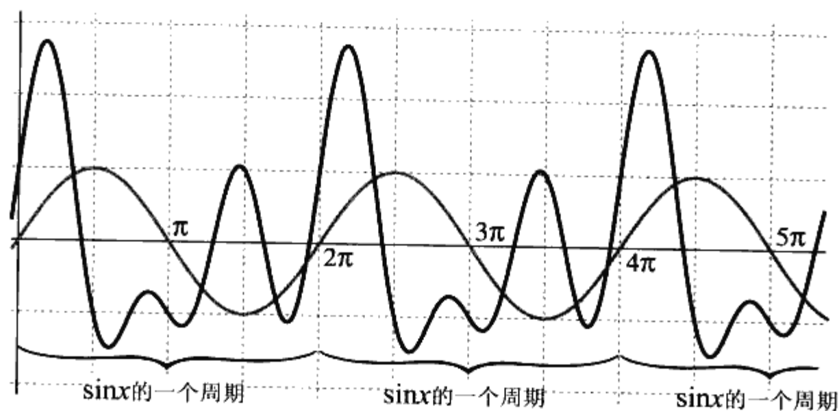
◆图6.21 \sin 2x + \sin 3x + \cos x 以 \sin x 的一个周期为基准
