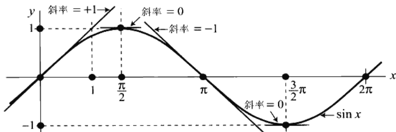
◆图3.14 y = \sin x 各点的切线的斜率
