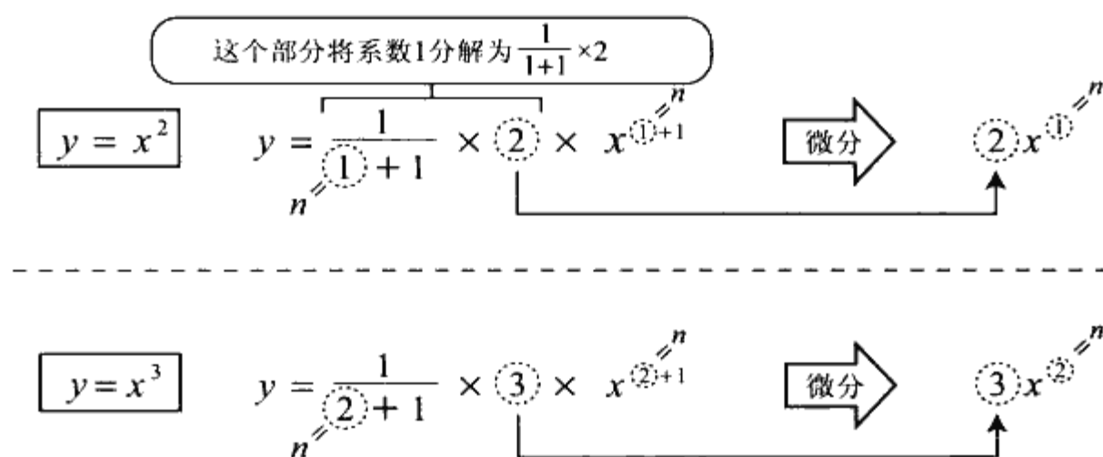
◆图 3.12 从积分的逆运算考虑 y = x^2 和 y = x^3 的微分：为了使系数仍保持为 1，乘以 2
