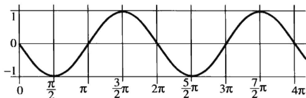
◆图 3.19 \cos 函数的导函数
