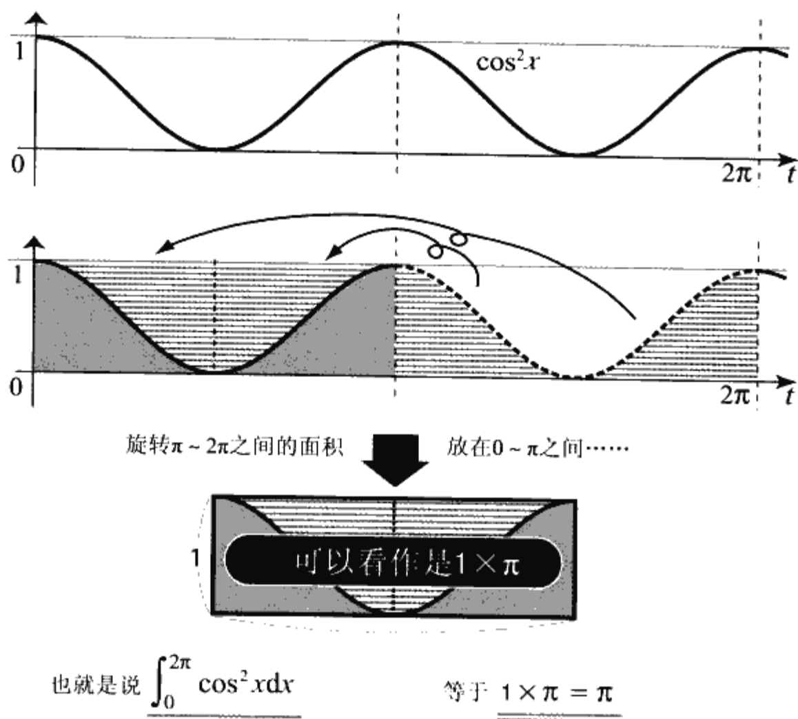
◆图 7.1 图形表示的 \cos^2 x 的积分结果
