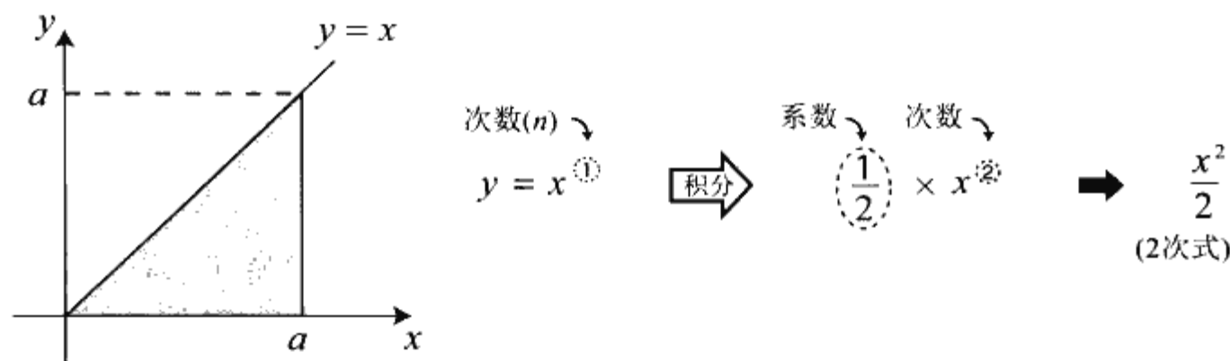
◆ 图 3.7 y=x 的积分
