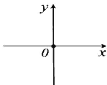
◆图6.3 相交成直角的 x 轴与 y 轴的图形
