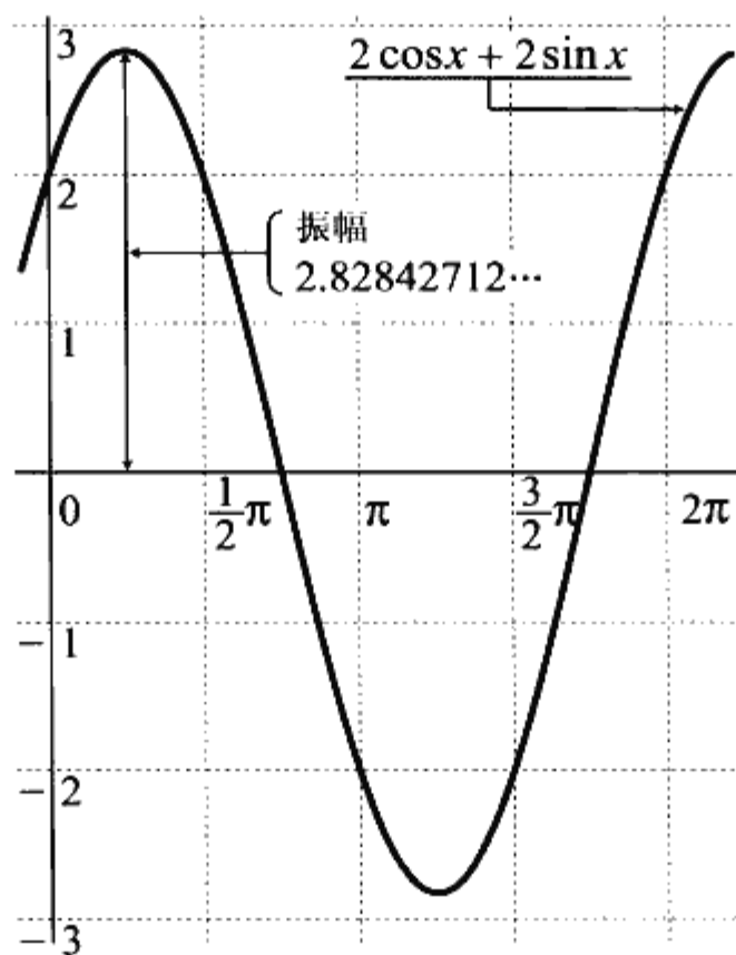
◆图 6.7 2\cos x + 2\sin x 的振幅
