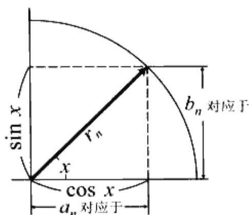
◆图7.3 表示频率成分的大小的图形
