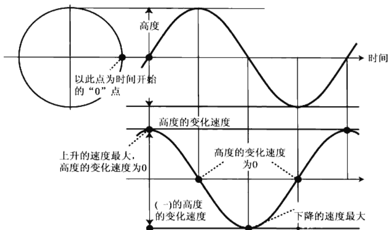
◆图3.17 观缆车的高度图和高度变化的速度图
