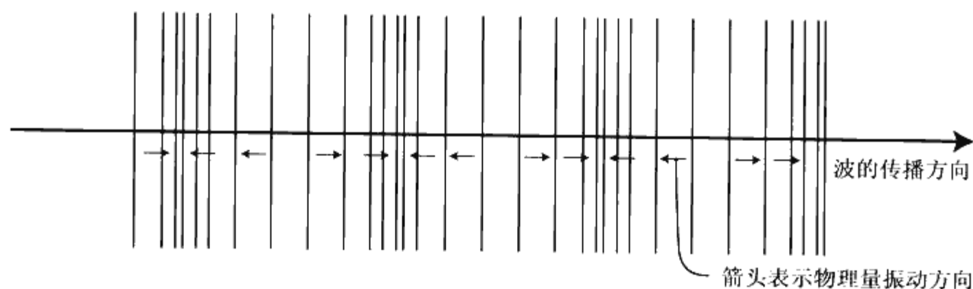
◆图1.3 纵波图形
