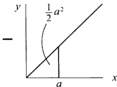
◆图 3.5 从 x = 0 到 x = b 的三角形面积中减去从 x = 0 到 x = a 的三角形面积
