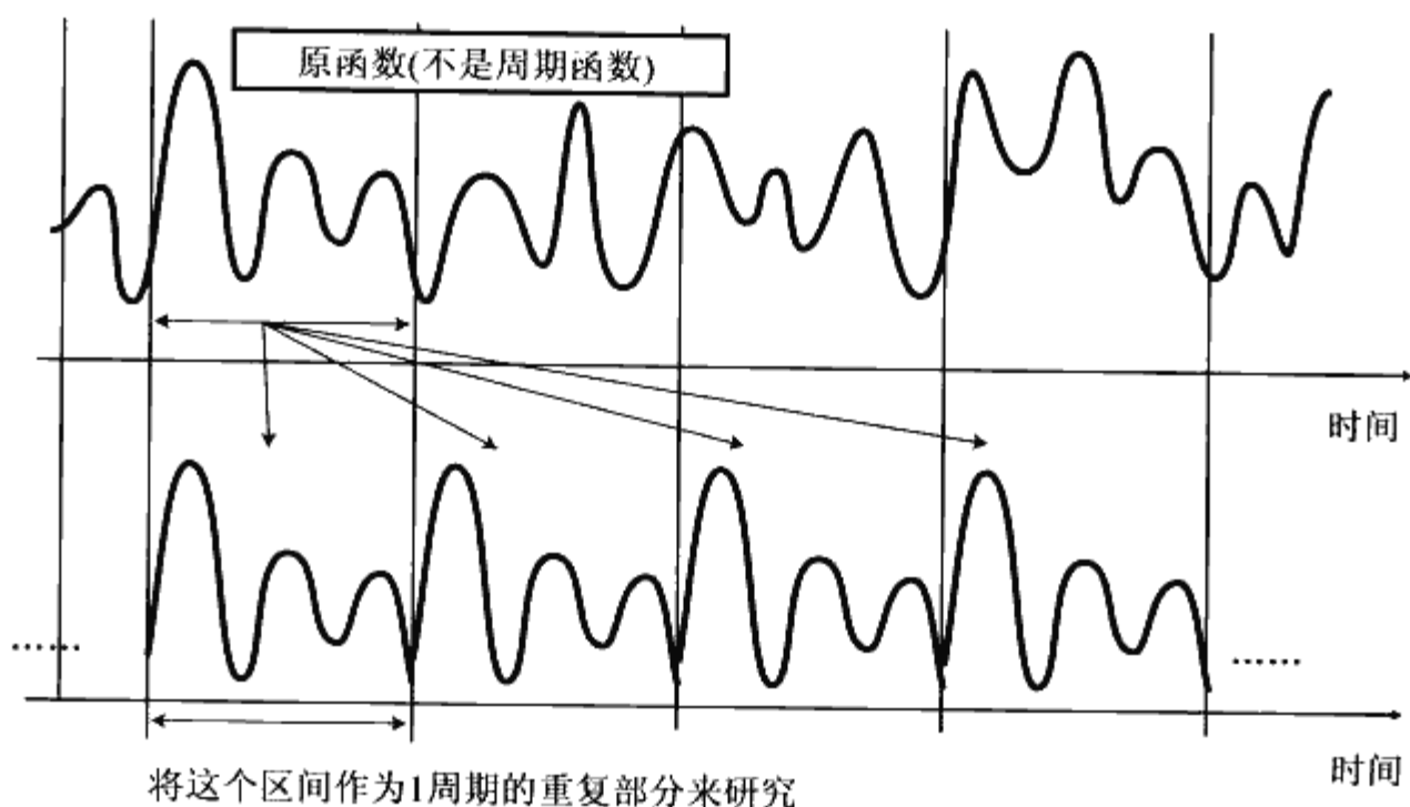
◆图6.22 将复杂波形作为周期函数来研究的方法
