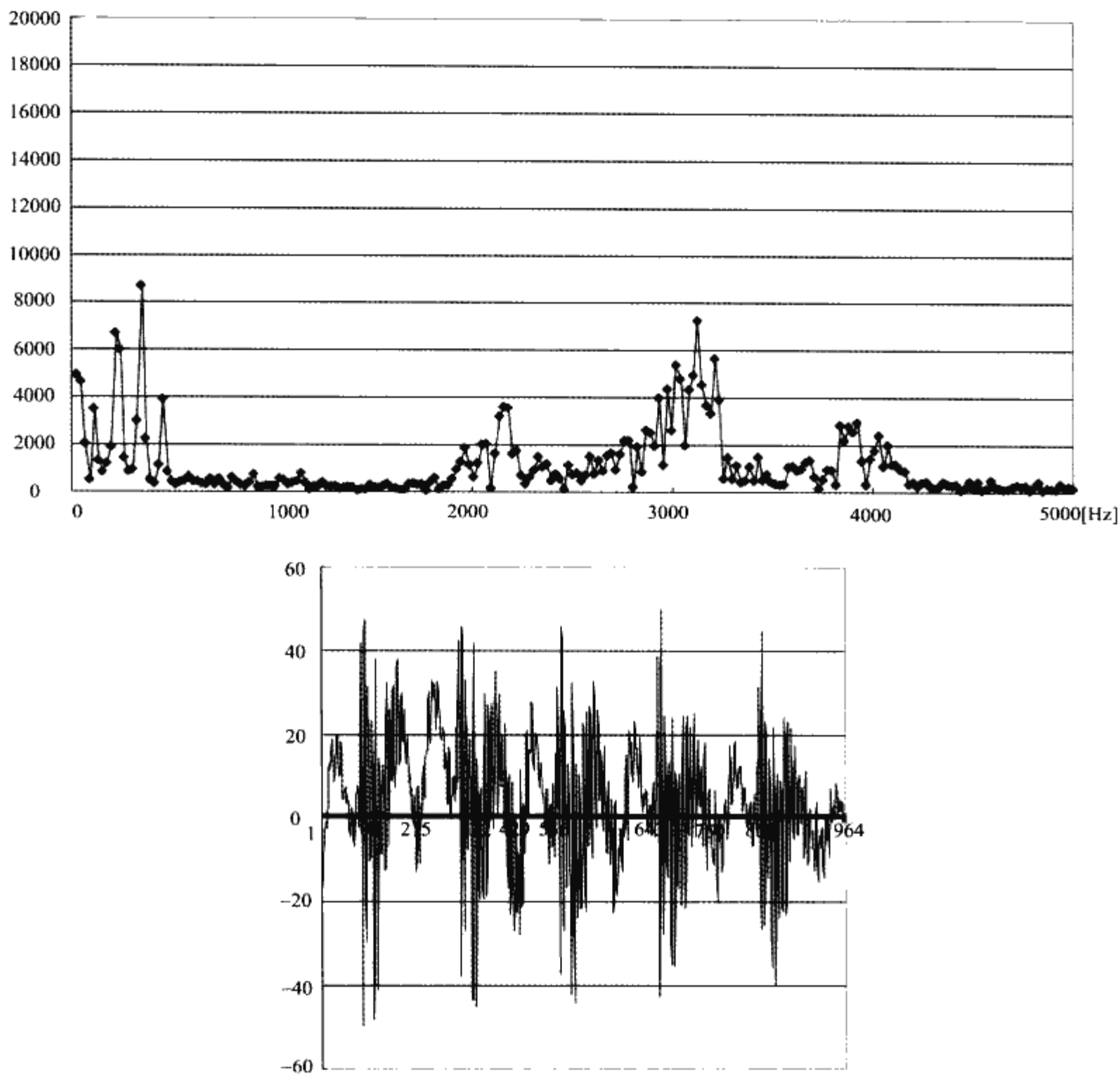
◆图7.17 “依”的频率谱与波形
