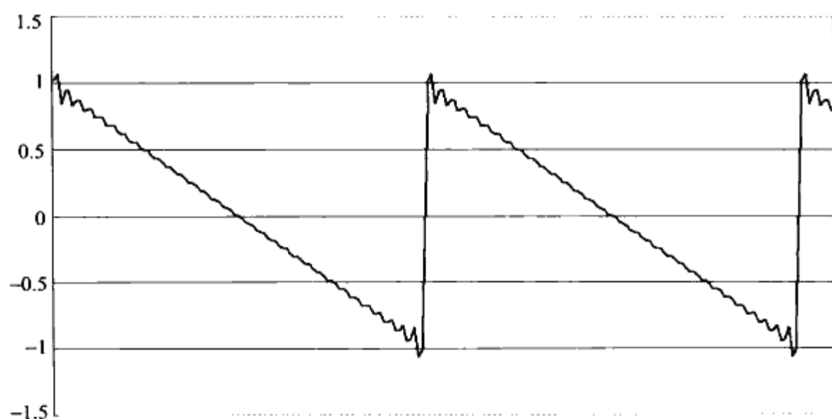
◆图 6.14 \sin 函数从 1 到 40 的依次累加的合成函数
