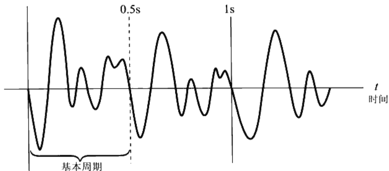
◆图1.13 基本周期
