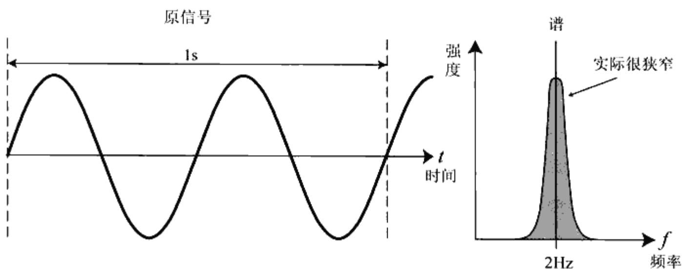
◆图 1.9 2Hz 信号转换为频率谱
