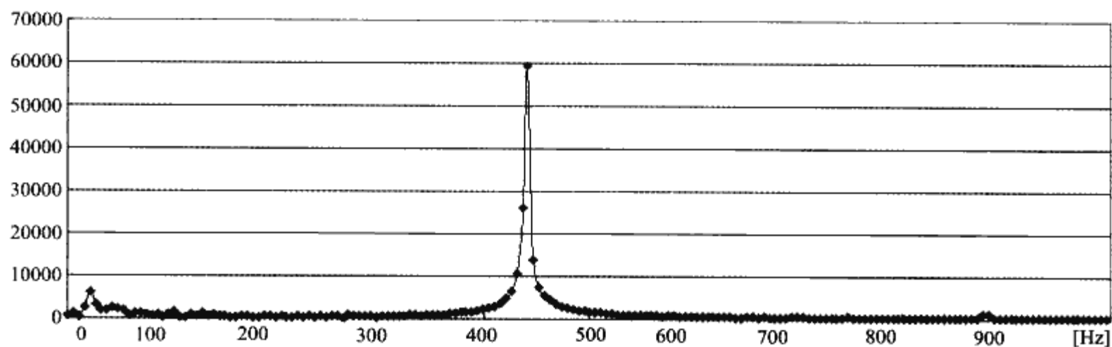
◆图7.9 音叉的频率谱
