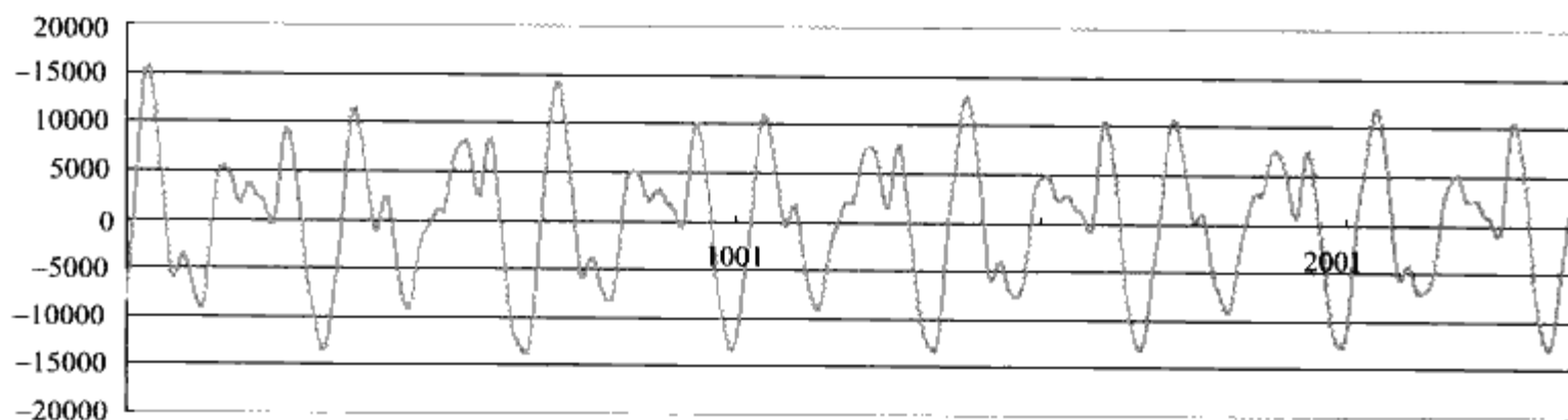
◆图 7.12 吉他的哆C、咪E、嗦G的波形
