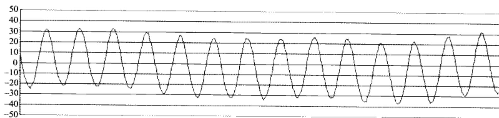
◆图7.8 音叉的波形
