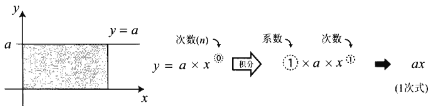
◆ 图 3.6 y=a 的积分
