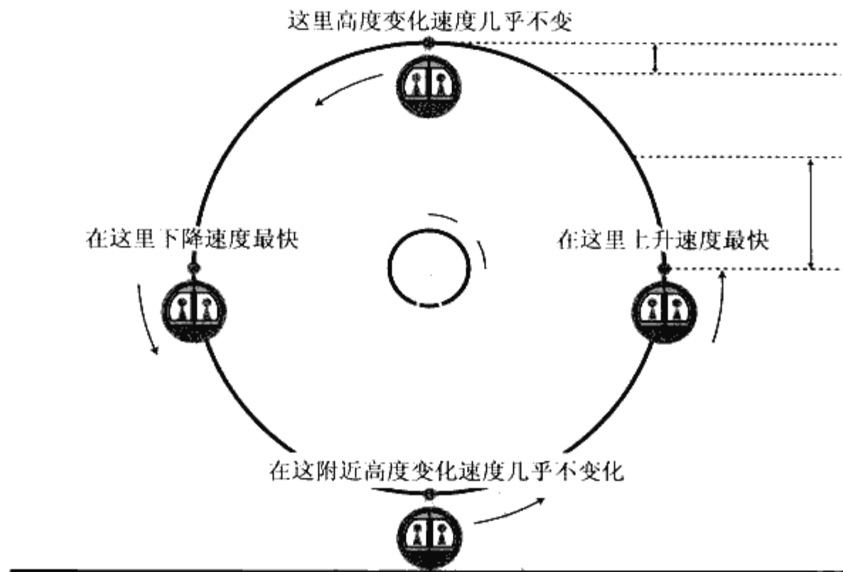
◆图 3.16 研究摩天轮的观缆车高度的变化情况
