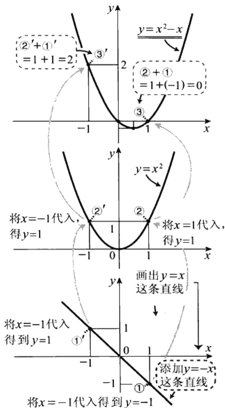
◆图 4.2 y=x^2 和 y=x 的减法运算
