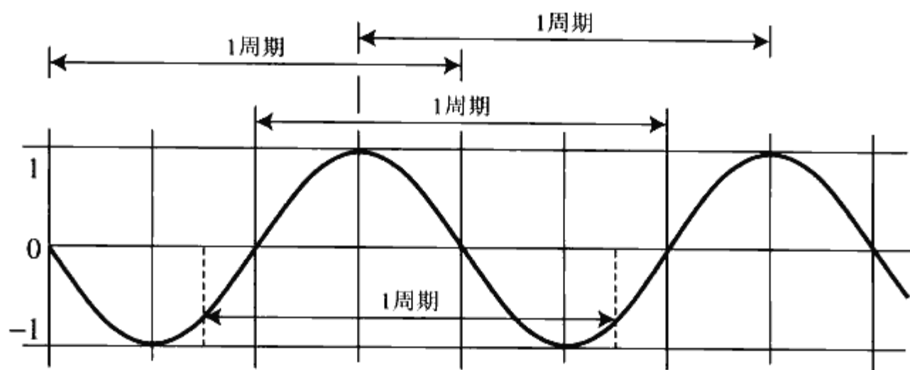
◆图1.8 1个周期的概念
