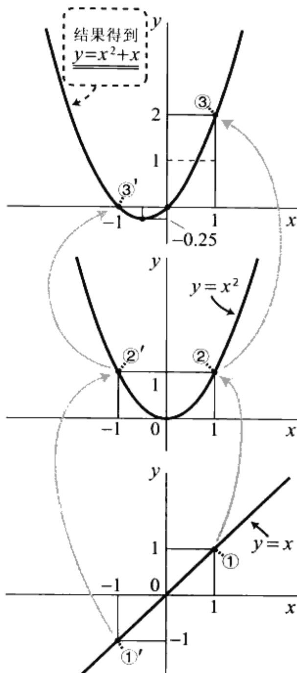
◆图 4.1 y=x^2 和 y=x 的加法运算
