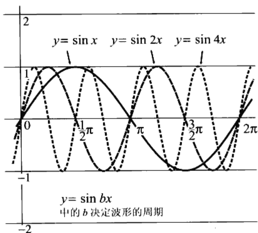
◆图 4.6 sin 前面和后面的数字与波形的关系
