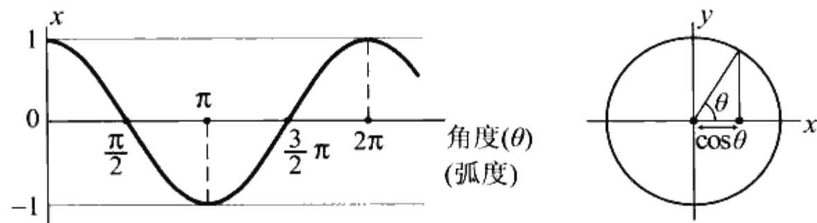
◆图2.3 余弦函数
