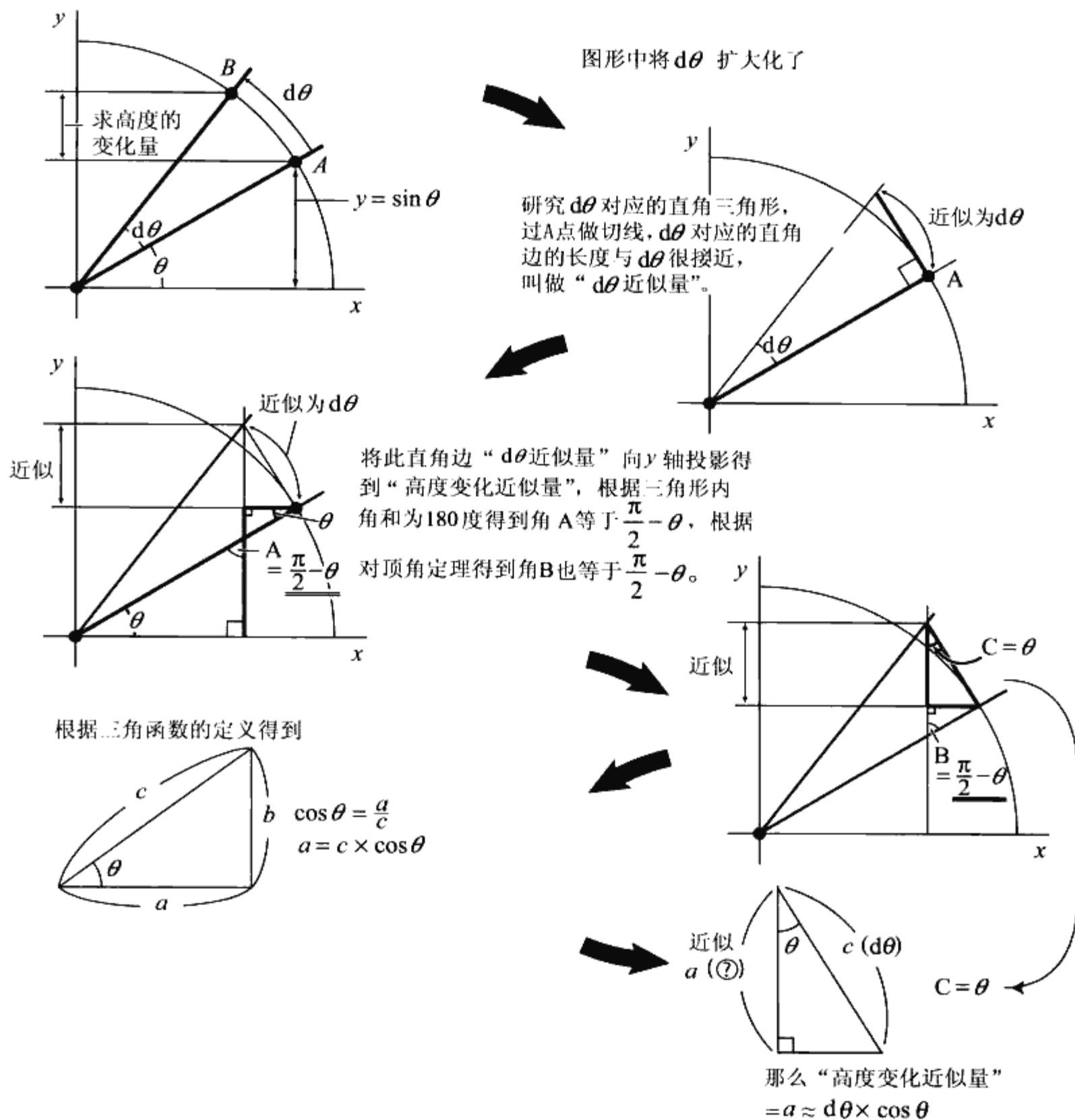
◆图 3.18 求高度 y 的变化
