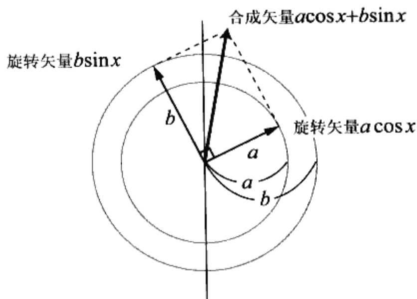
◆图 6.5 两正交旋转矢量 a \cos x 与 b \sin x 的合成的概念
