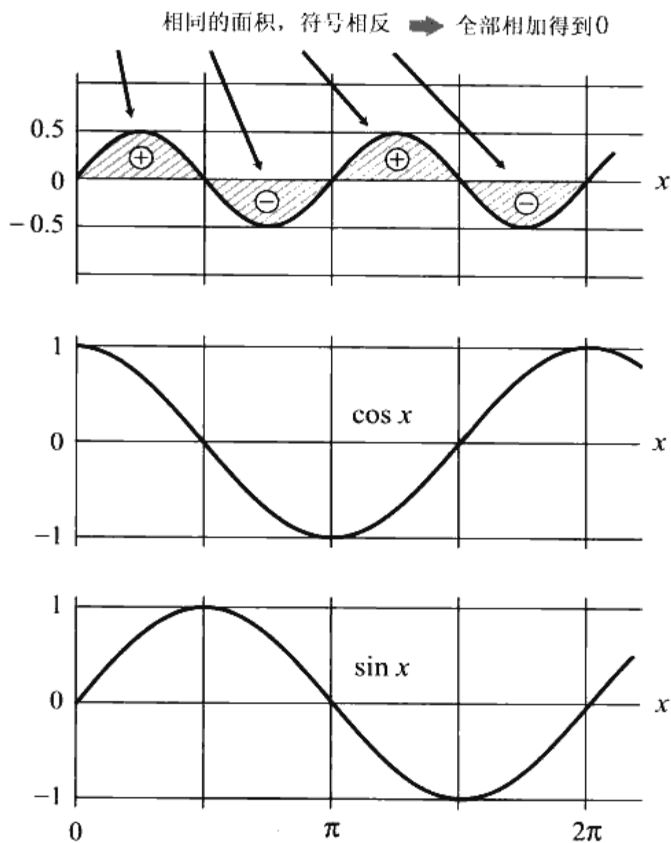
◆图5.1 \sin x 与 \cos x 的积的定积分
