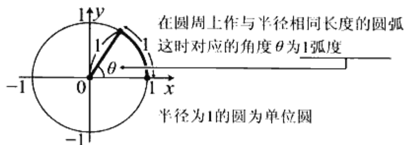
◆图2.1 单位圆中的弧度概念
