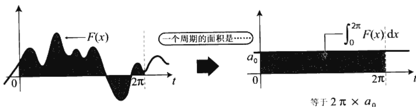
◆图 7.2 用图形说明复杂波形 F(x) 的积分结果
