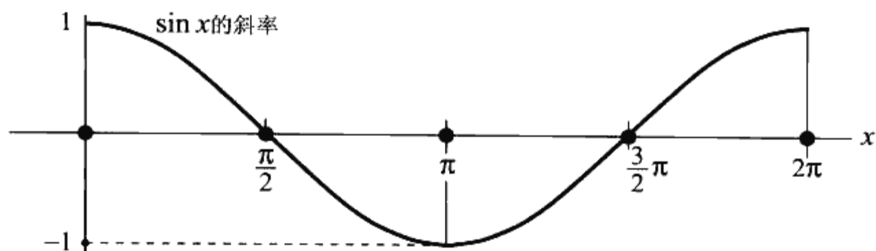
◆图 3.15 y = \sin x 的斜率的变化
