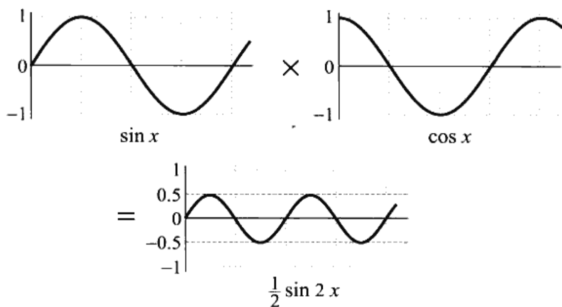
◆图 4.5 y = \sin x 与 y = \cos x 的积
