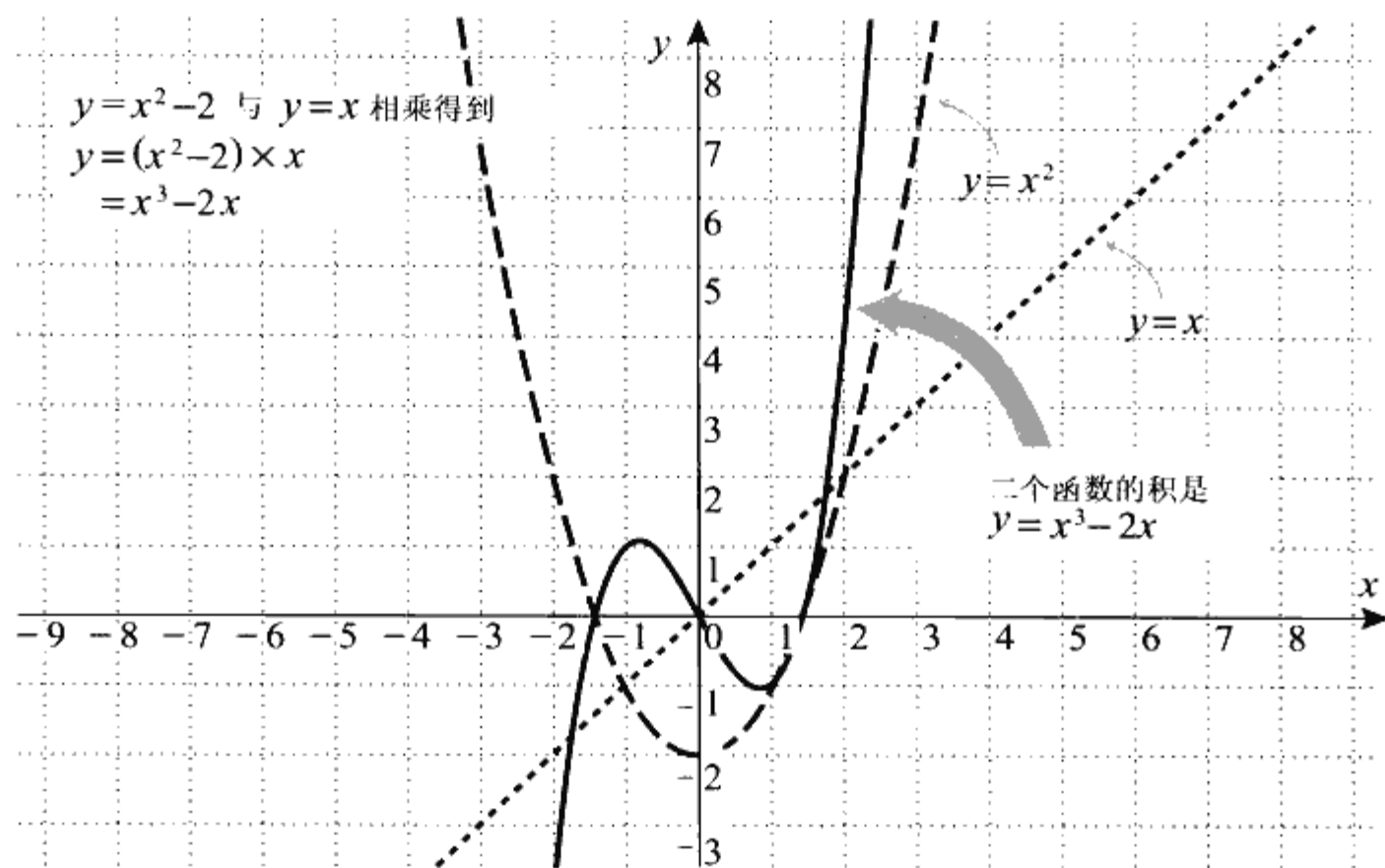
◆图 4.3 y = x^2 - 2 和 y = x 的积
