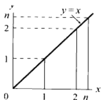
◆图3.3 y=x 的图形
