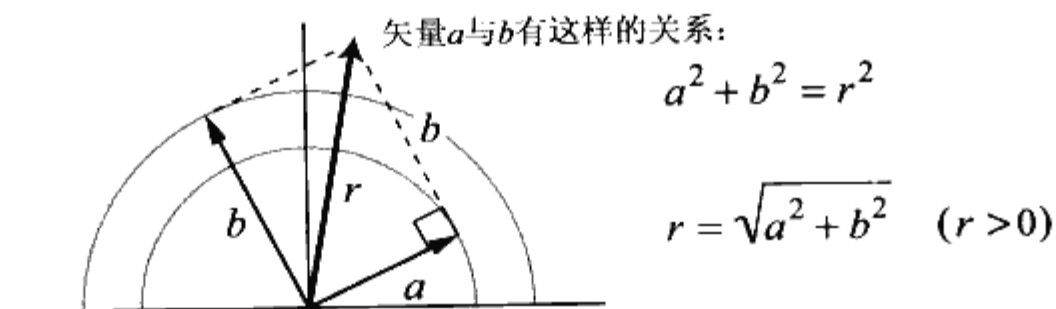
◆图6.6 矢量合成中毕达哥拉斯定理的应用
