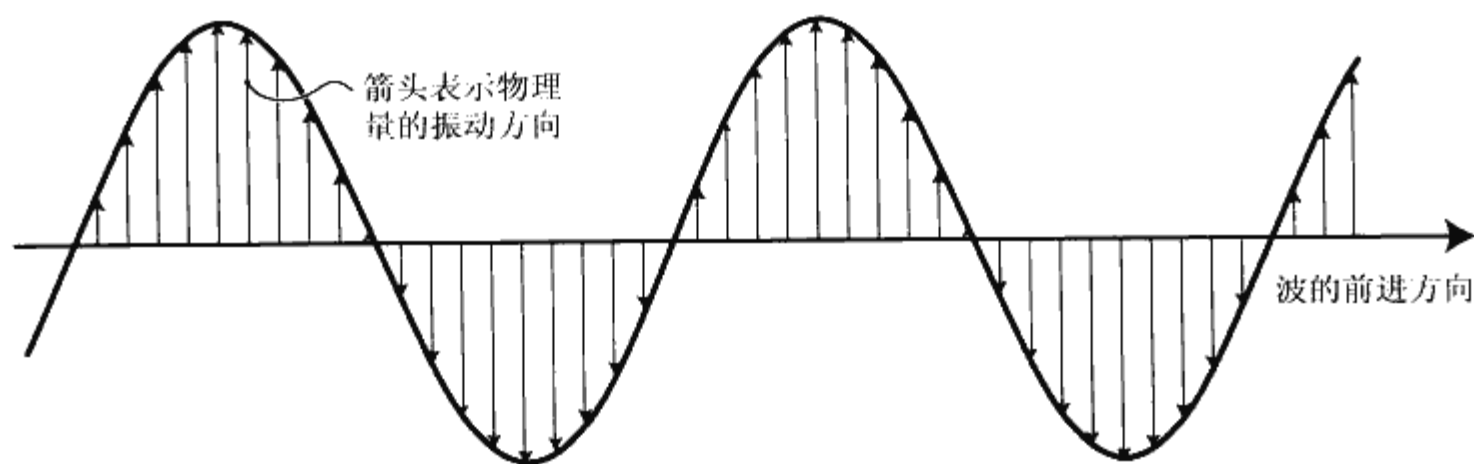
◆图1.2 横波图
