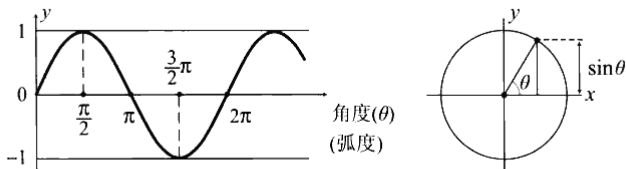
◆图2.2 正弦函数的概念
