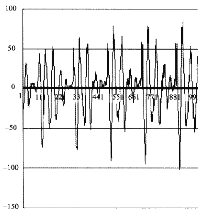
◆图7.20 “喔”的频率谱与波形
