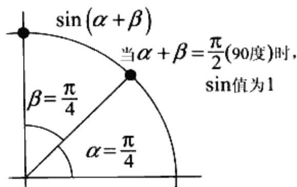
◆图 4.7 \sin(\alpha + \beta) 的图象
