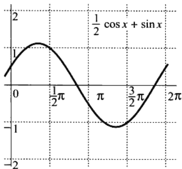
◆图6.1 \frac{1}{2}\cos x + \sin x 的波形的相位
