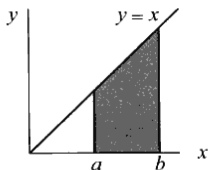
◆图 3.4 求 x = a 到 x = b 的梯形面积
