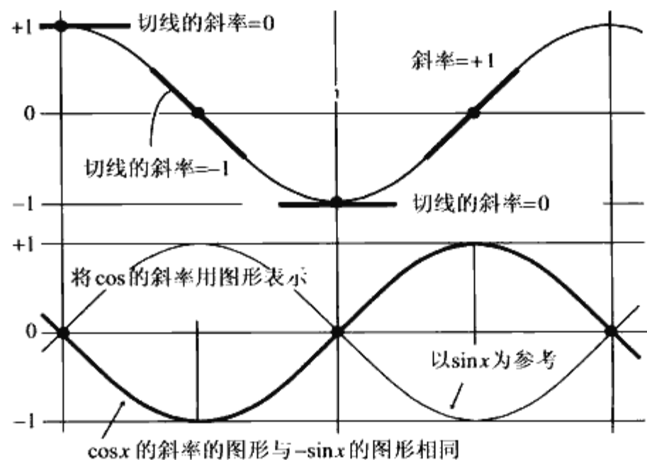
◆图 3.20 y = \cos x 的导函数的研究方法
