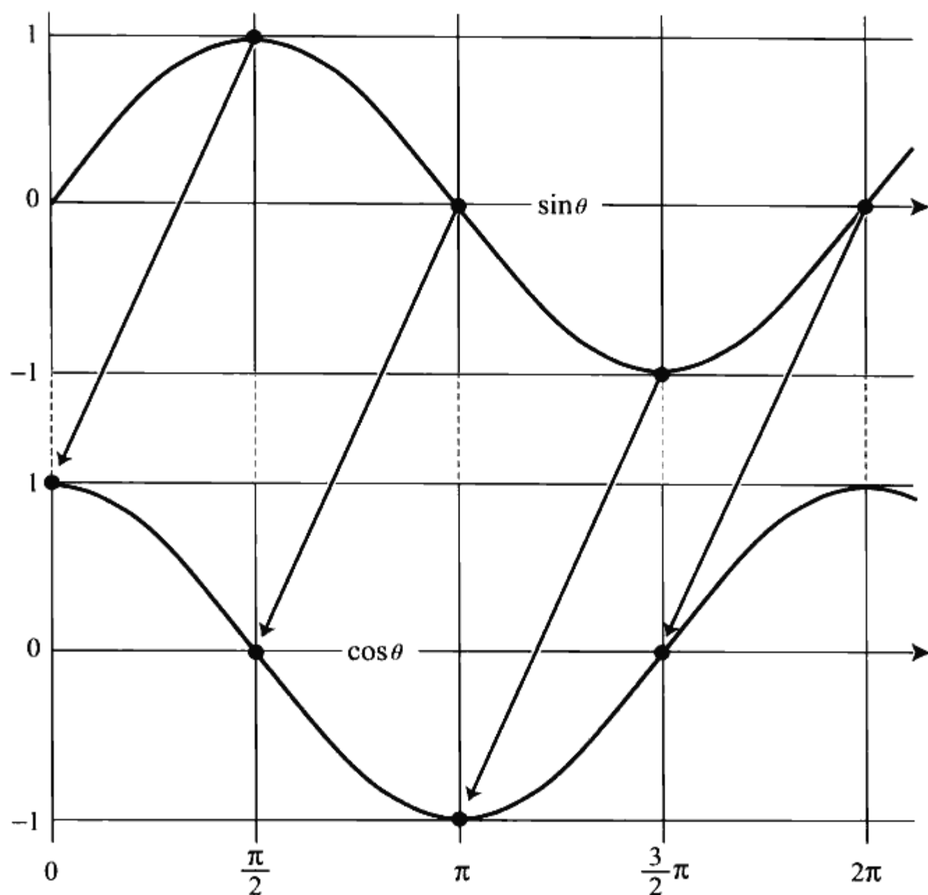
◆图 2.4 \sin \theta 与 \cos \theta
