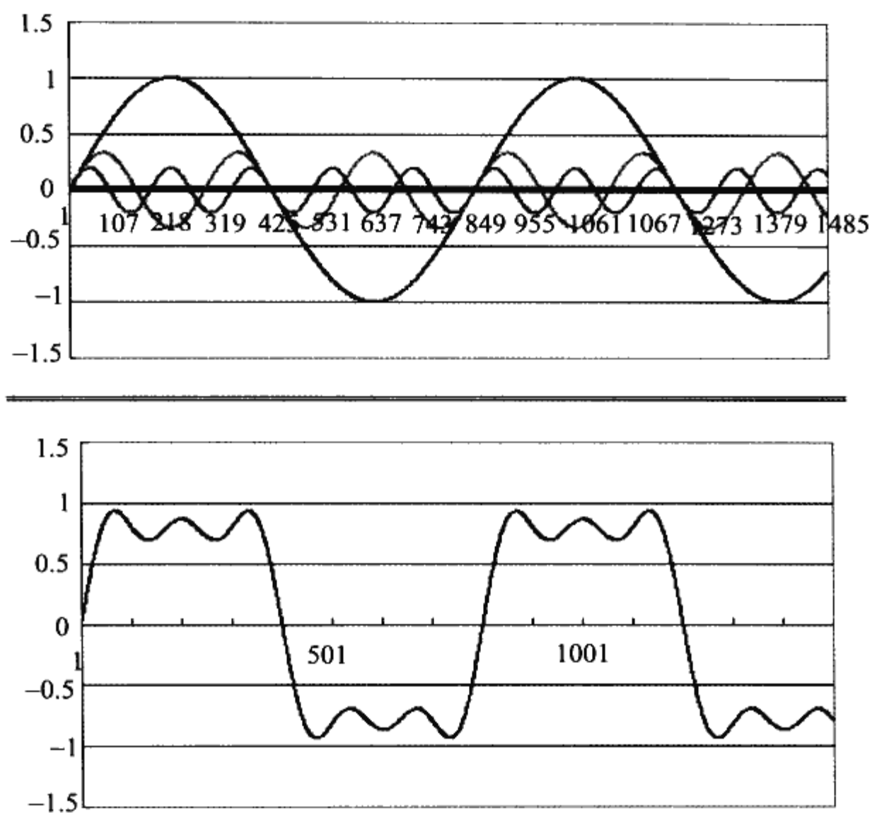
◆图 6.15 奇数次的 sin 函数从 1 到 5 的依次累加的合成函数
