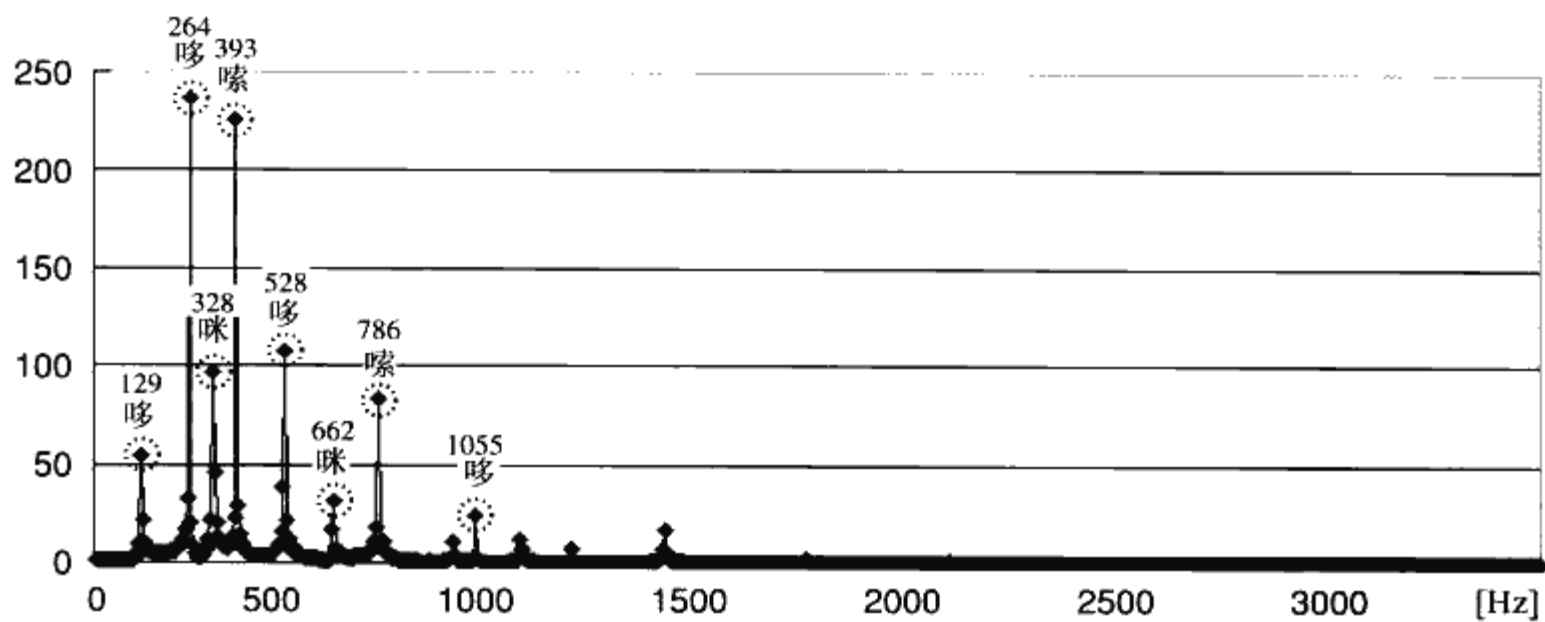
◆图 7.13 哆C、咪E、嗦G音的频率谱中的主要峰值的频率
